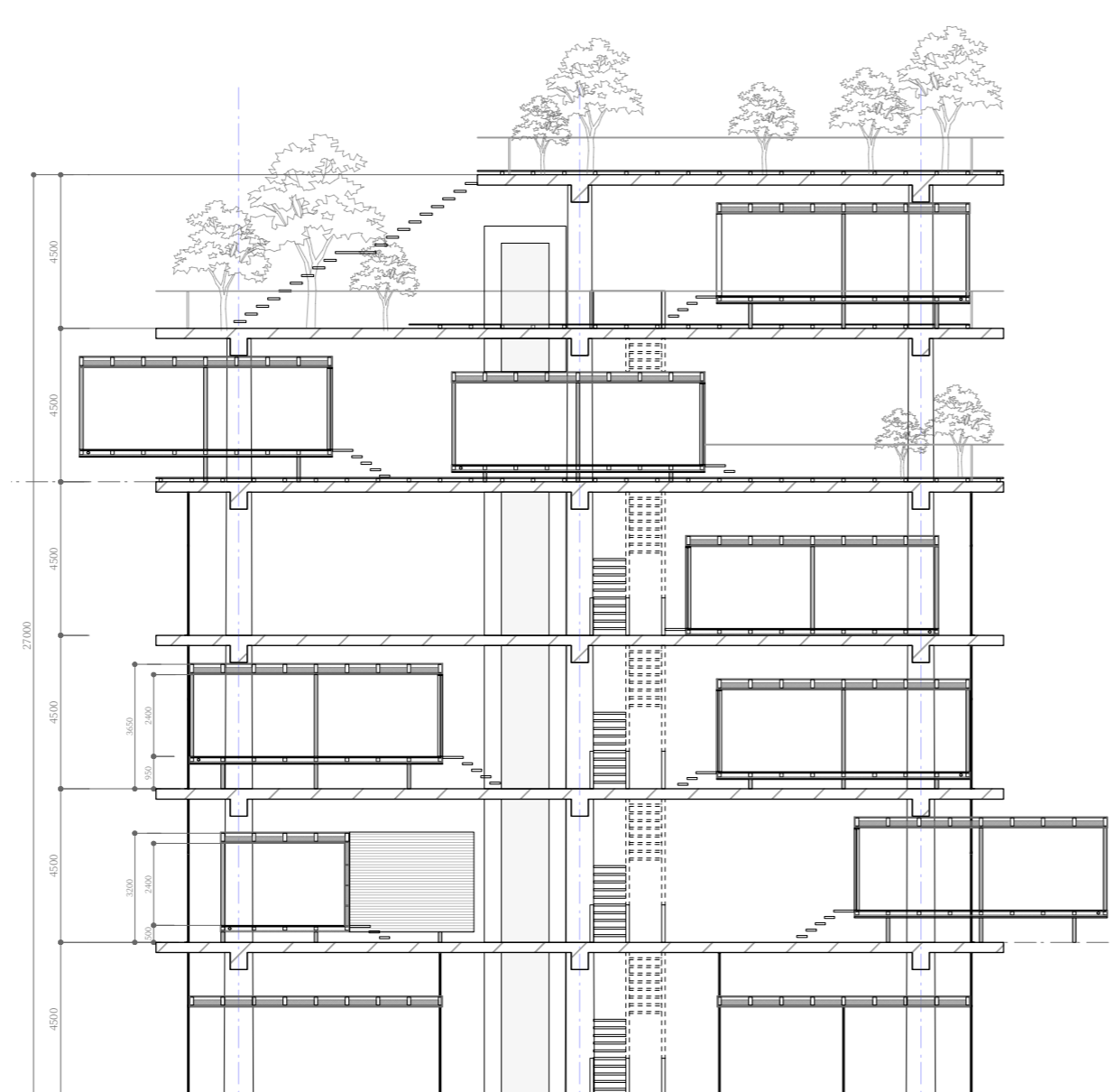
断面図 S=1/200
