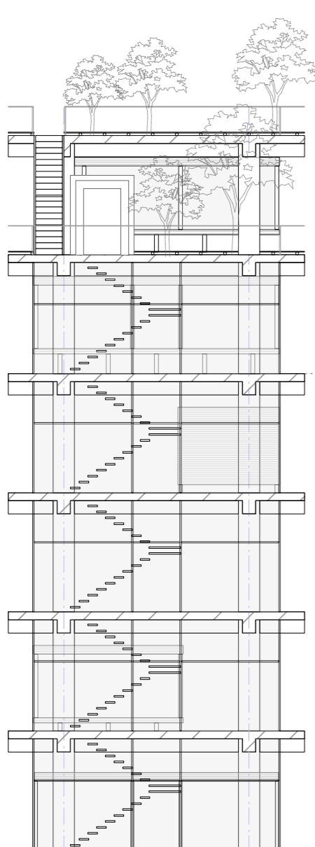
南立面図 S=1/200
