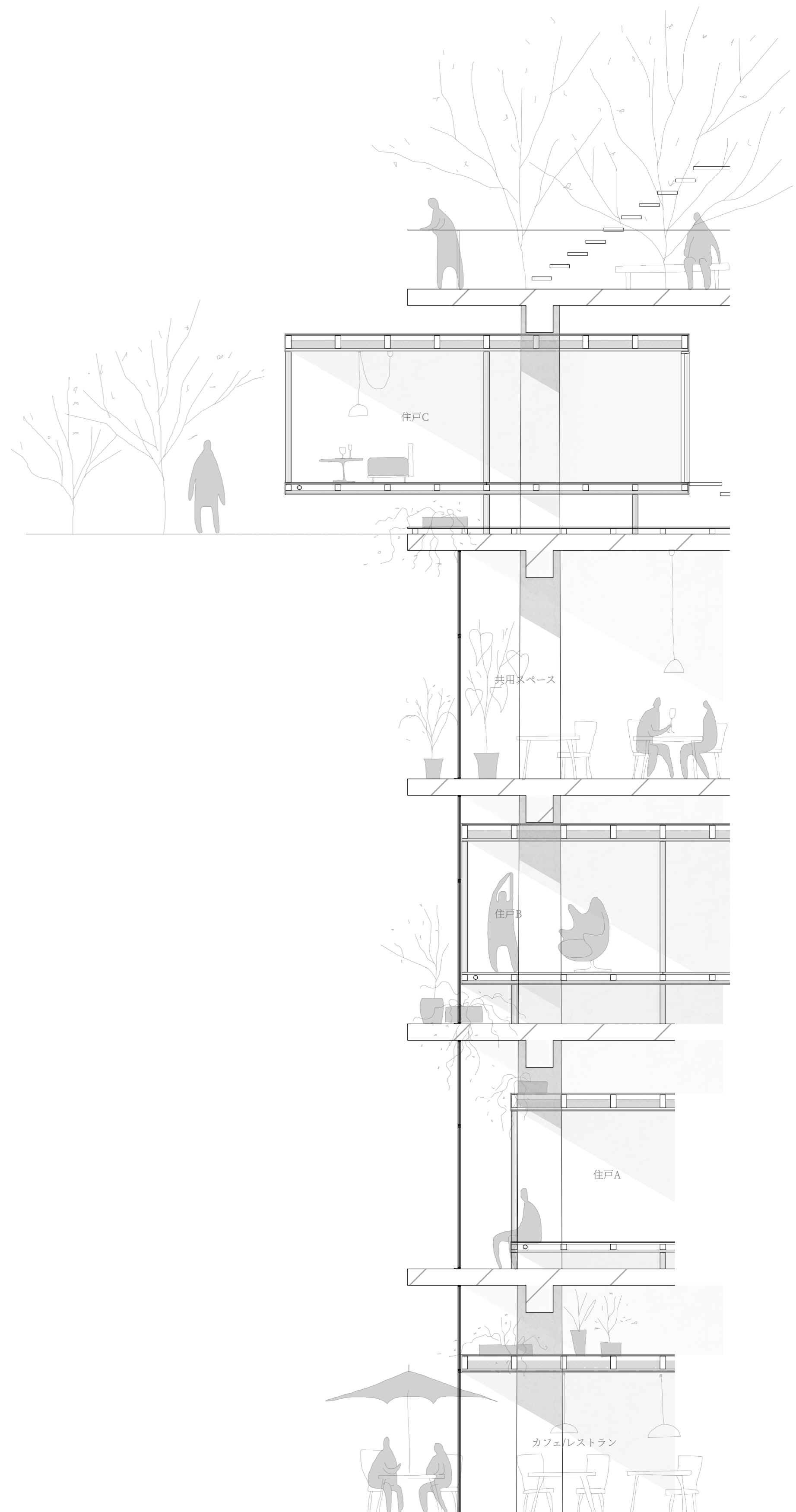
断面詳細図 S=1/60
